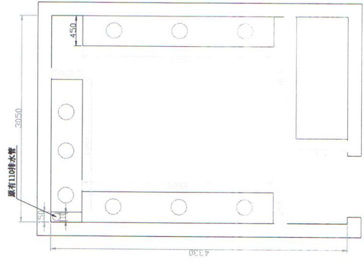
平面布置图
