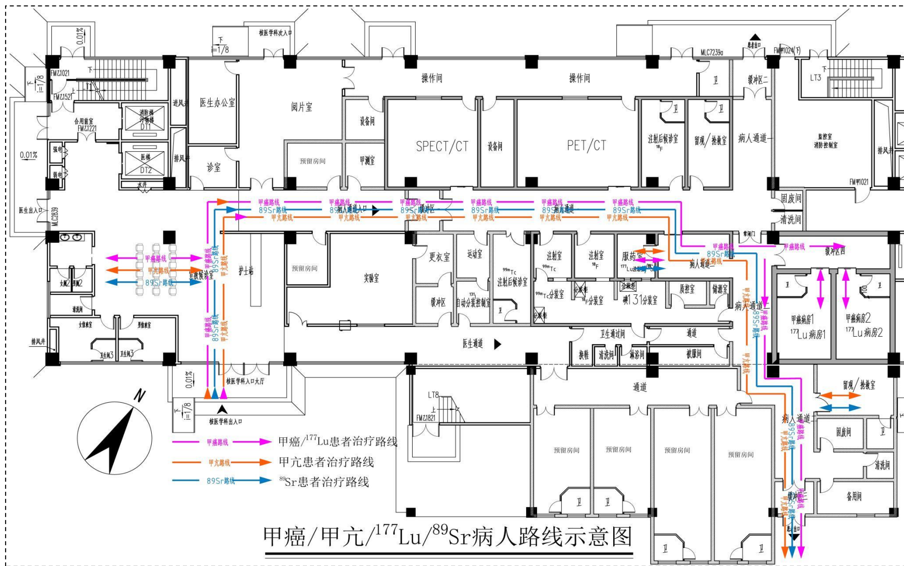
图 9-12 核医学科接受治疗项目人员活动路径示意图
