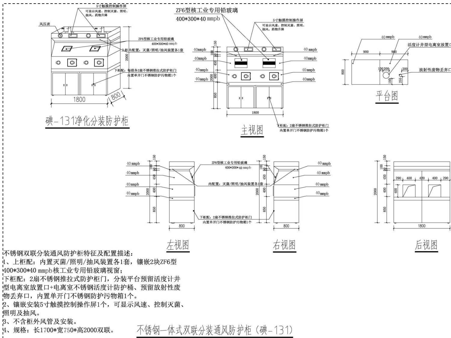
图 10-6 碘分装柜设计示意图
