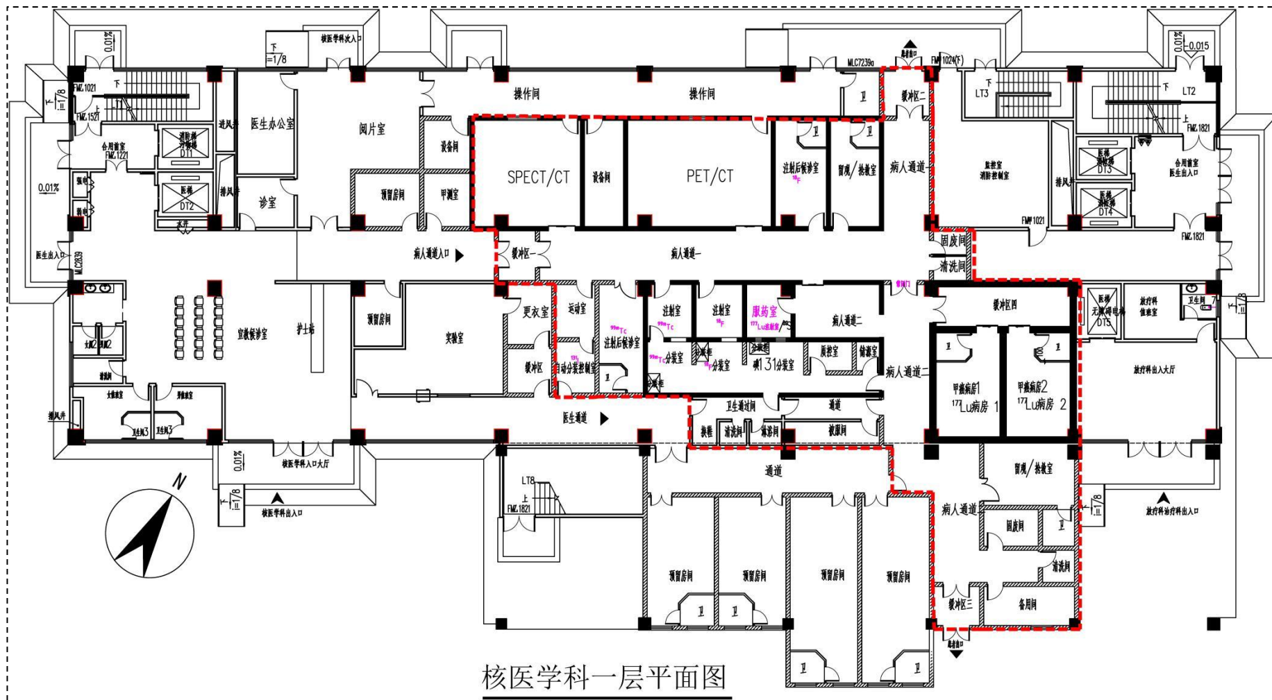
图 1-11 致远楼一层拟建核医学科平面布置示意图
