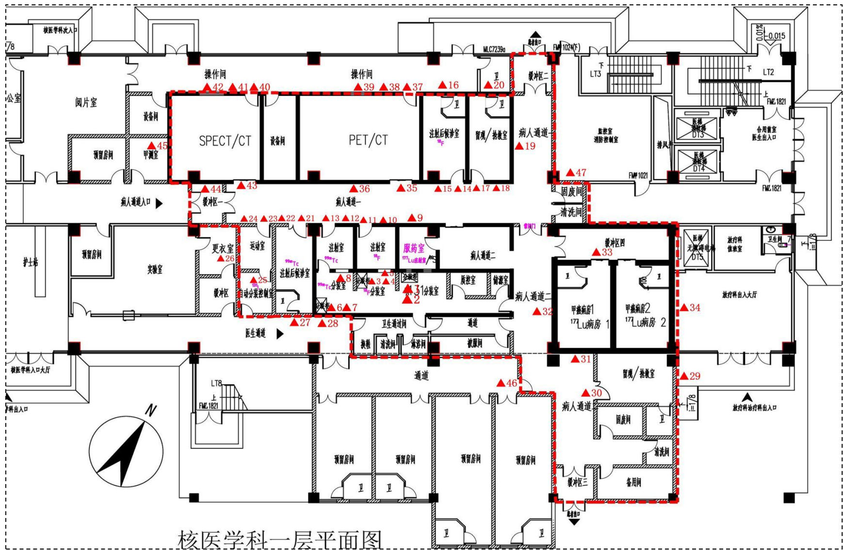
图 11-1 一层核医学科场所关注点示意图
