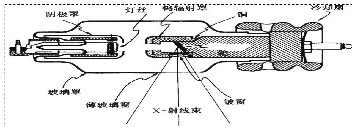
图 9-8 X 射线管结构原理图
