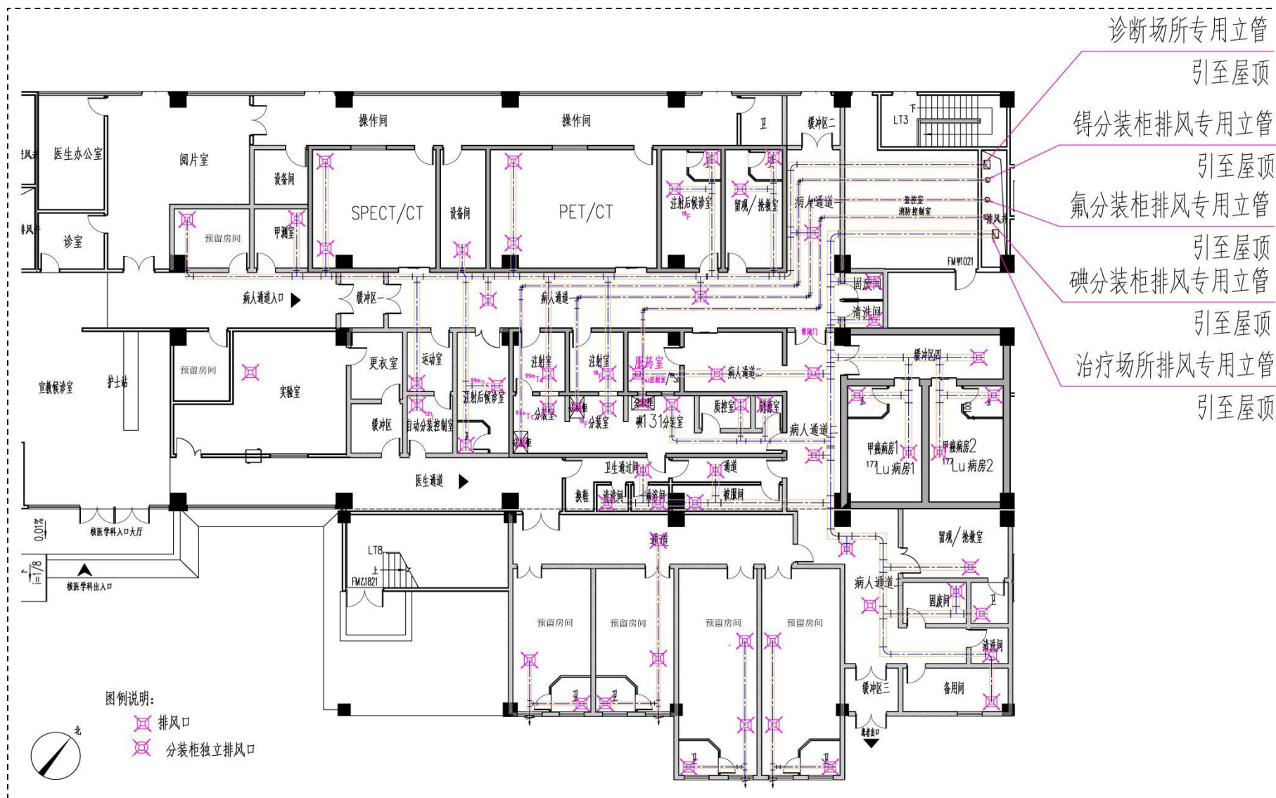
图 10-15 核医学工作场所排风路线示意图
