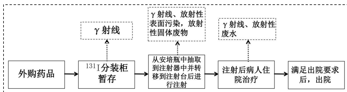
图 9-7 ^{177}\text{Lu} 治疗项目工作流程及产污环节
