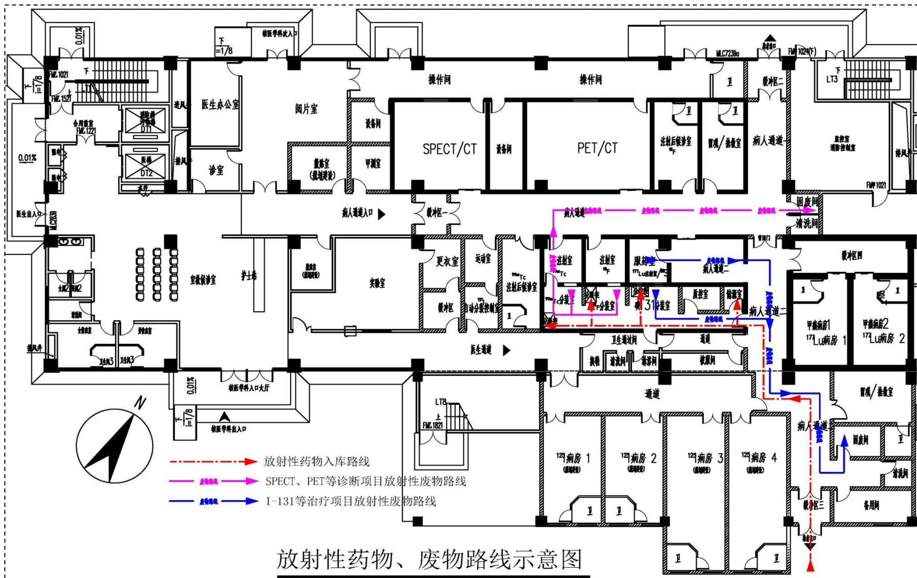
图 9-11 放射性药物、废物路径示意图
