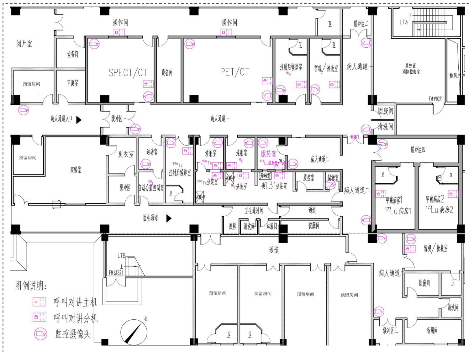
图 10-2 核医学工作场所视频监控及对讲系统布局示意图
