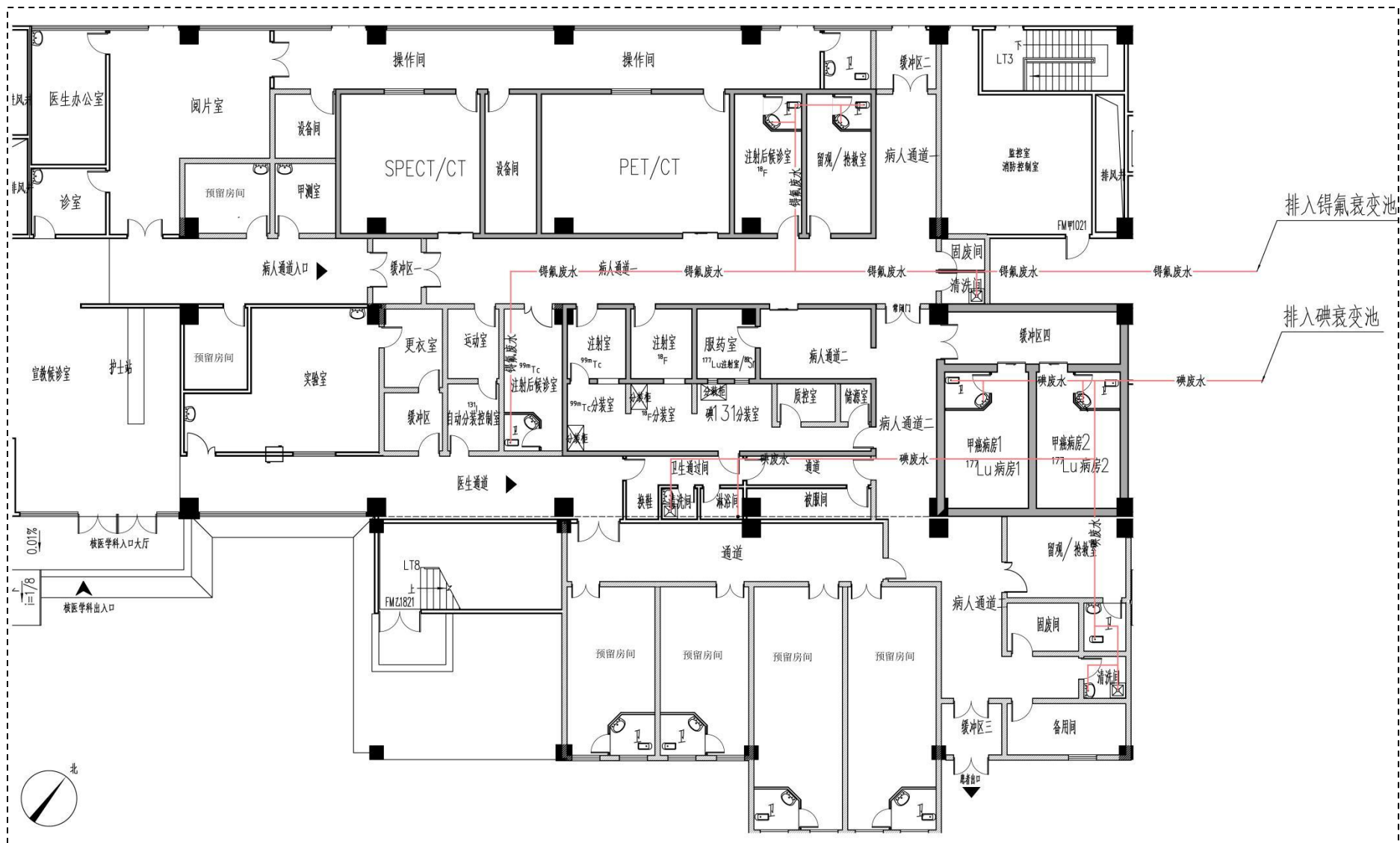
图 10-11 核医学工作场所放射性废水排放路线示意图
