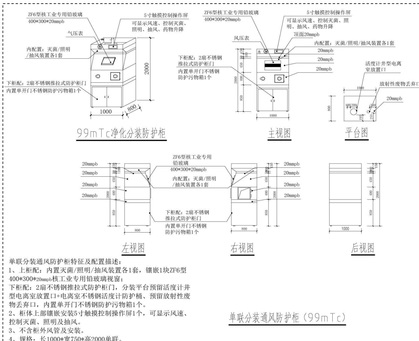
图 10-5 锝分装柜设计示意图
