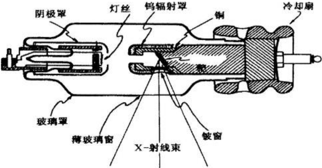
图 9-1 X 射线管结构原理图
