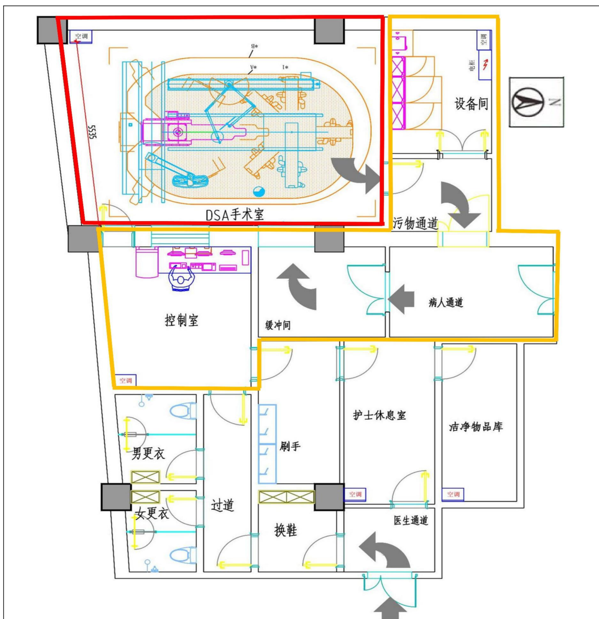
图 10-1 DSA 机房平面布置图
