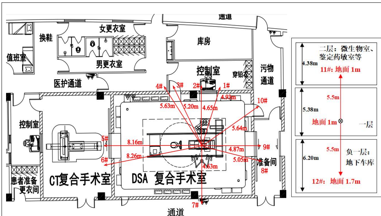
图13.3-2 1#门诊医技楼一层急诊中心DSA+CT复合手术室关注点示意图
