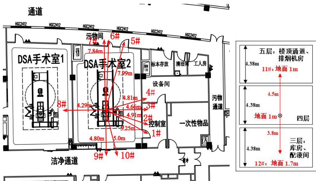
图13.3-5 1#门诊医技楼四层手术部DSA2机房关注点示意图
