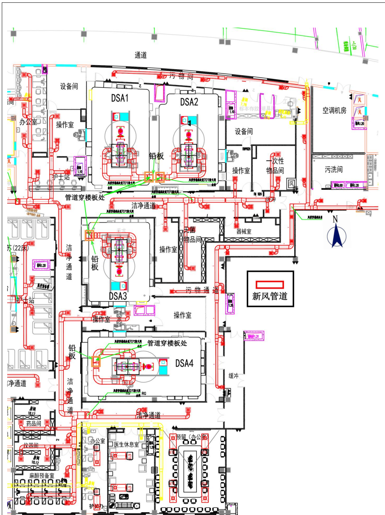
图 10.3-21 1#门诊医技楼四层手术部 DSA 机房新风管道布置示意图
