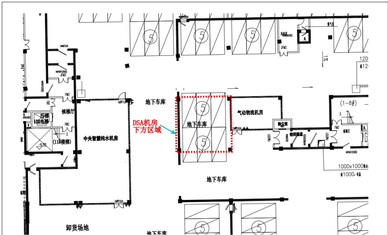
图 10.3-3 1#门诊医技楼一层放射科 DSA 机房对应楼下平面布置图
