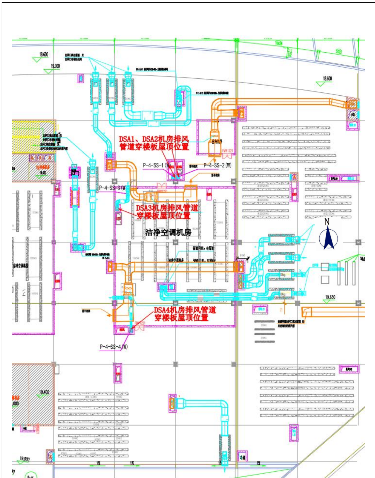
图 10.3-22 1#门诊医技楼四层手术部 DSA 机房屋顶排风管道出口示意图
