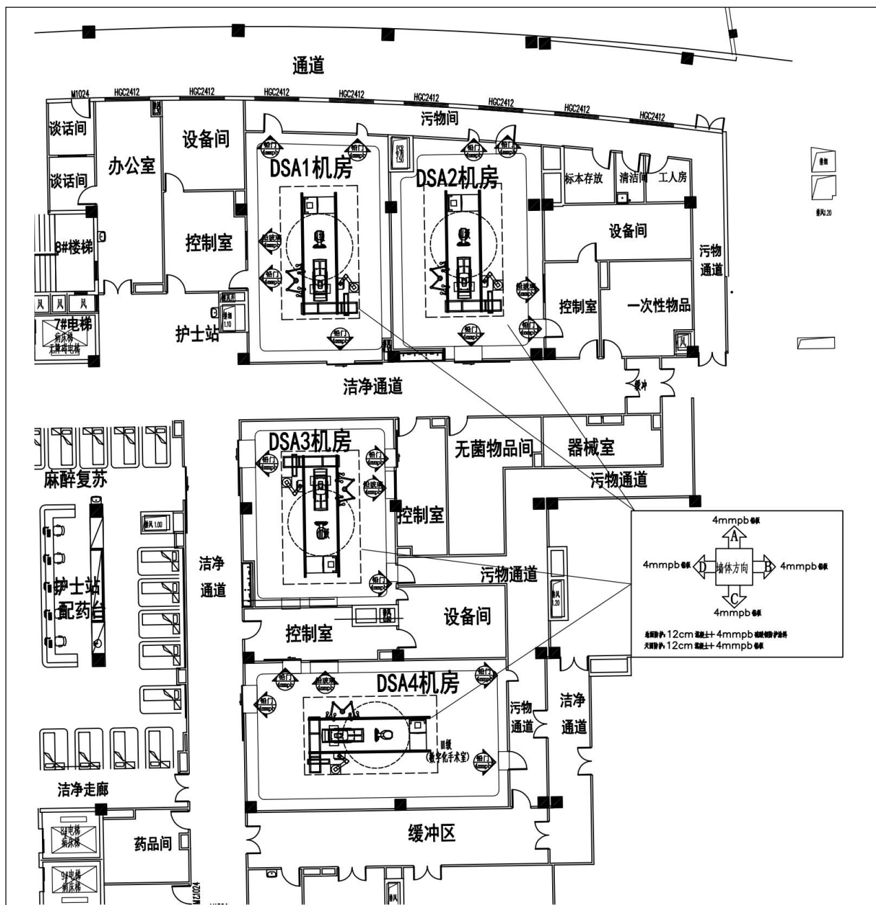
图10.3-16 1#门诊医技楼四层手术部DSA机房屏蔽防护设计示意图
