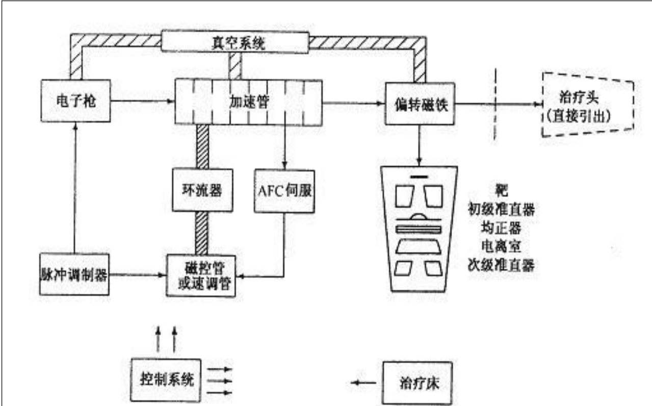
图 9.2-1 典型应用直线加速器内部结构框图
