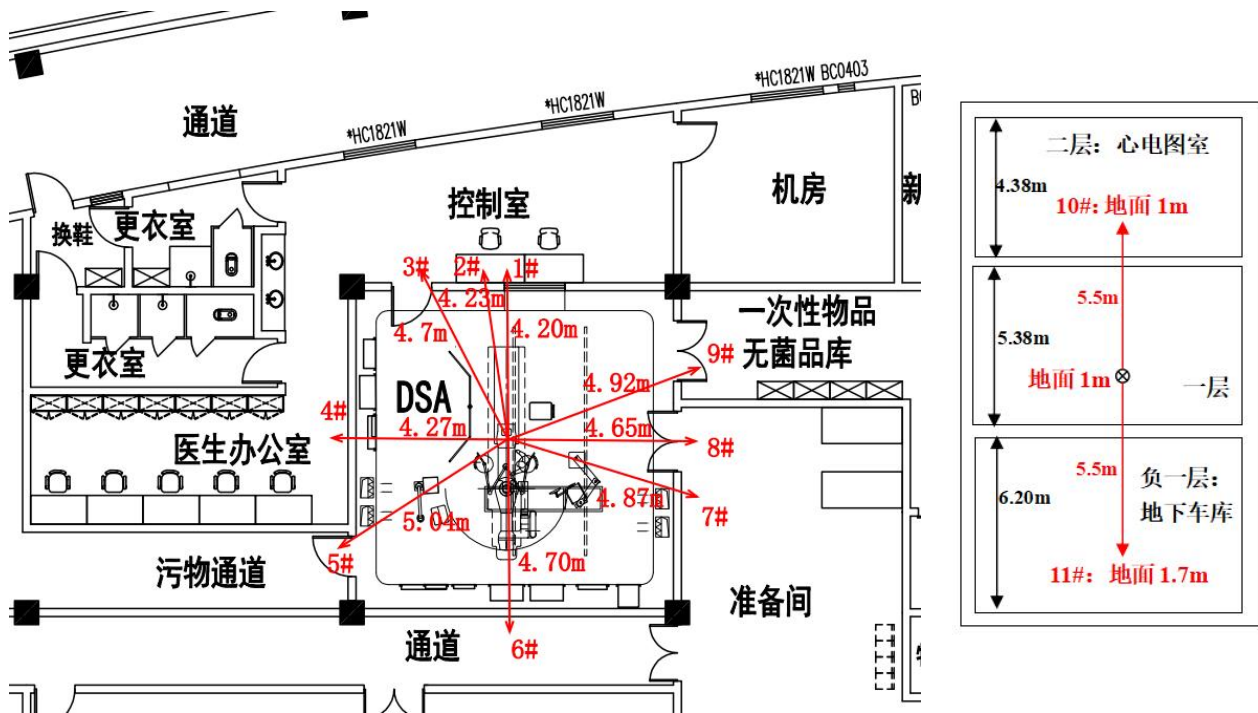
图 13.3-1 1#门诊医技楼一层放射科 DSA 机房关注点示意图
