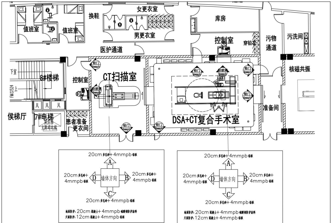
图10.3-14 1#门诊医技楼一层急诊中心DSA+CT复合手术室屏蔽防护设计示意图
