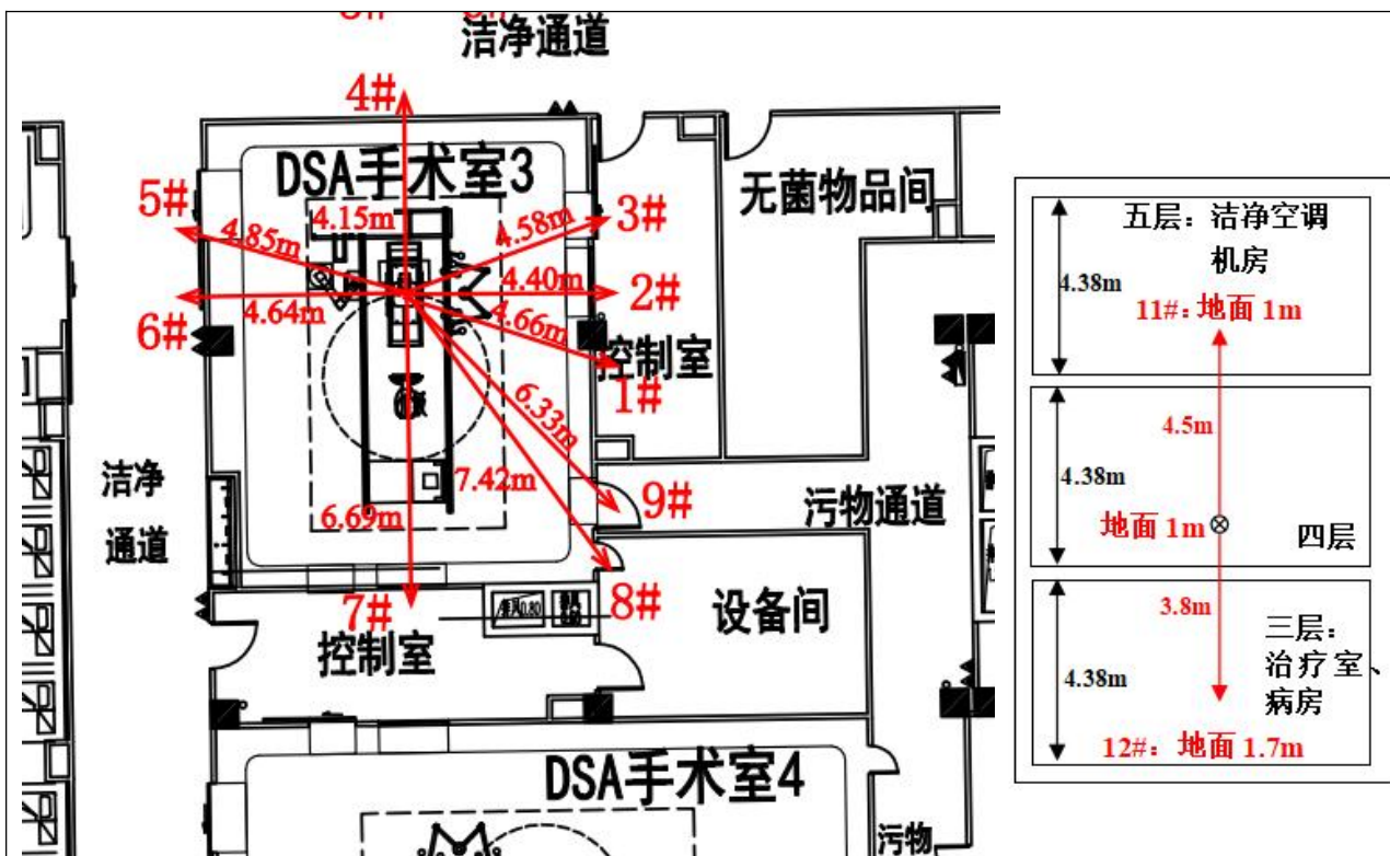
图13.3-6 1#门诊医技楼四层手术部DSA3机房关注点示意图
