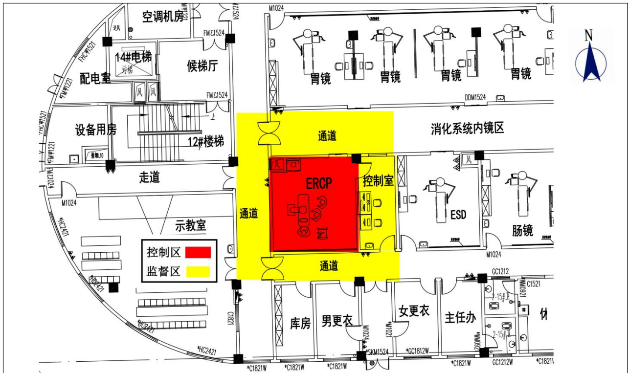
图10.3-10 1#门诊医技楼二层内镜中心ERCP机房工作场所分区示意图
