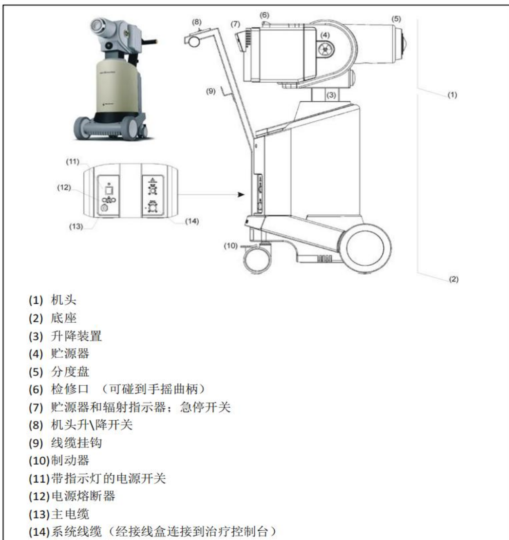
图 9.2-5 常见后装机结构示意图
