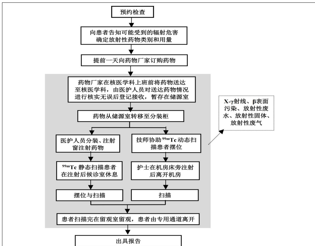
图 9.1-1 SPECT/CT 检查工作流程及产污环节示意图 ( ^{99m}\text{Tc} 放射性药物显像)
