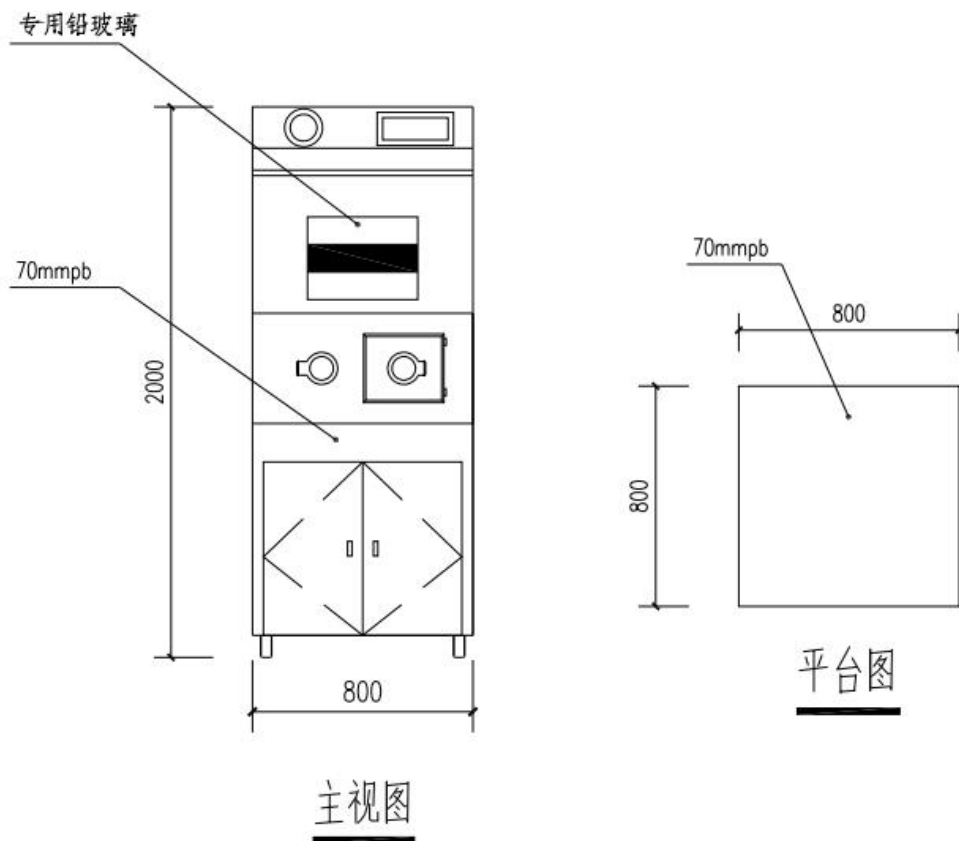
单联分装通风防护柜示意图（氟18）
