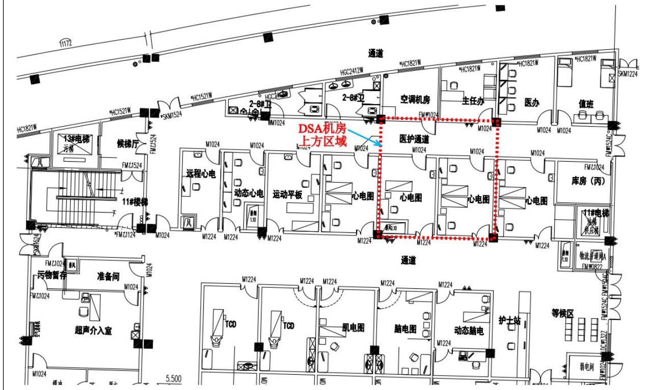
图 10.3-2 1#门诊医技楼一层放射科 DSA 机房对应楼上平面布置图
