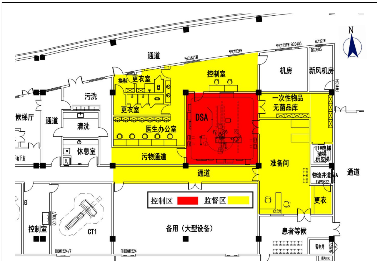
图10.3-1 1#门诊医技楼一层放射科DSA机房工作场所分区示意图
