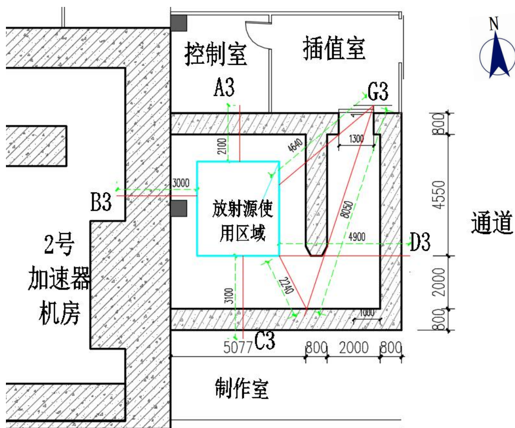
图11.2-3 后装机机房周围关注点平面示意图
