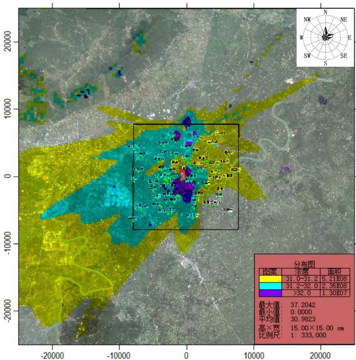
图4.2-23 正常排放 NO 2 叠加后保证率日平均质量浓度分布图 (单位: μg/m 3 )
