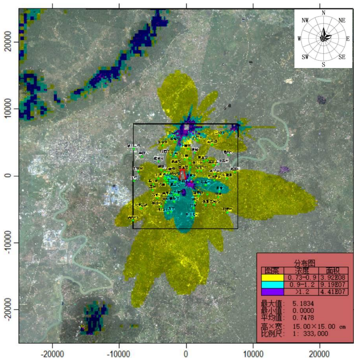
图4.2-36 正常排放 H 2 S 叠加后小时平均质量浓度分布图 (单位: μg/m 3 )
