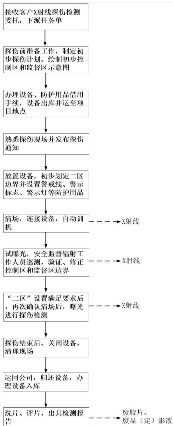
图9-5 探伤工作流程图
