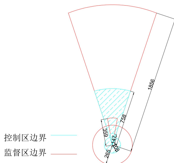
图 11-1 2005 型射线机分区示意图
