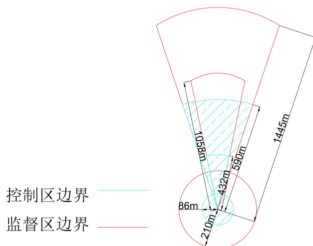
图 11-3 3505 型射线机控制区、监督区划分示意图
