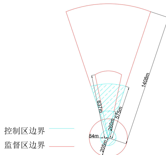
图 11-2 2505 型射线机分区示意图
