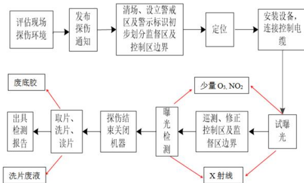
图 9-5 探伤项目工作流程示意图
