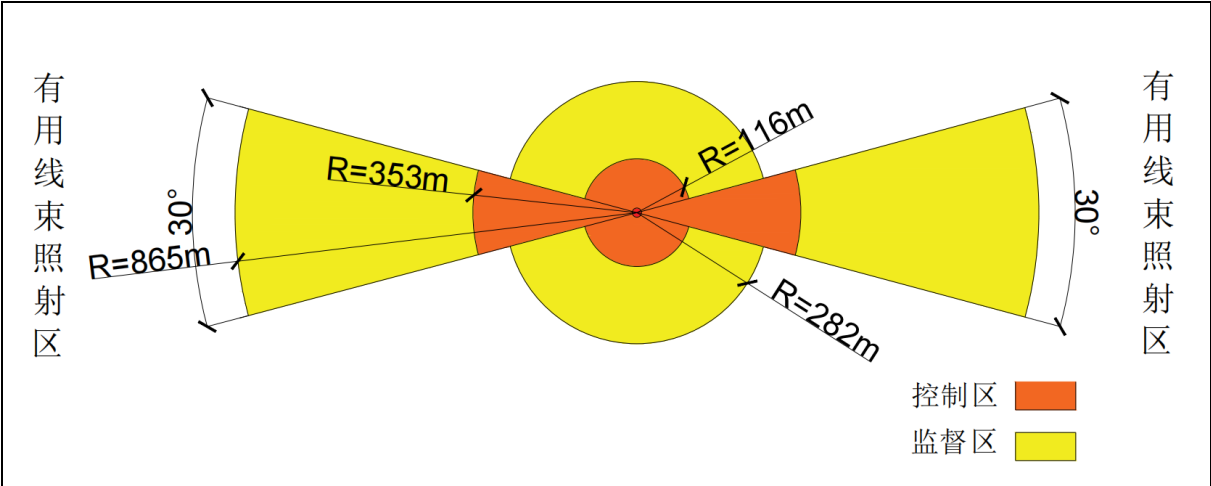
图 10-4 周向机监督区和控制区范围平面示意图
