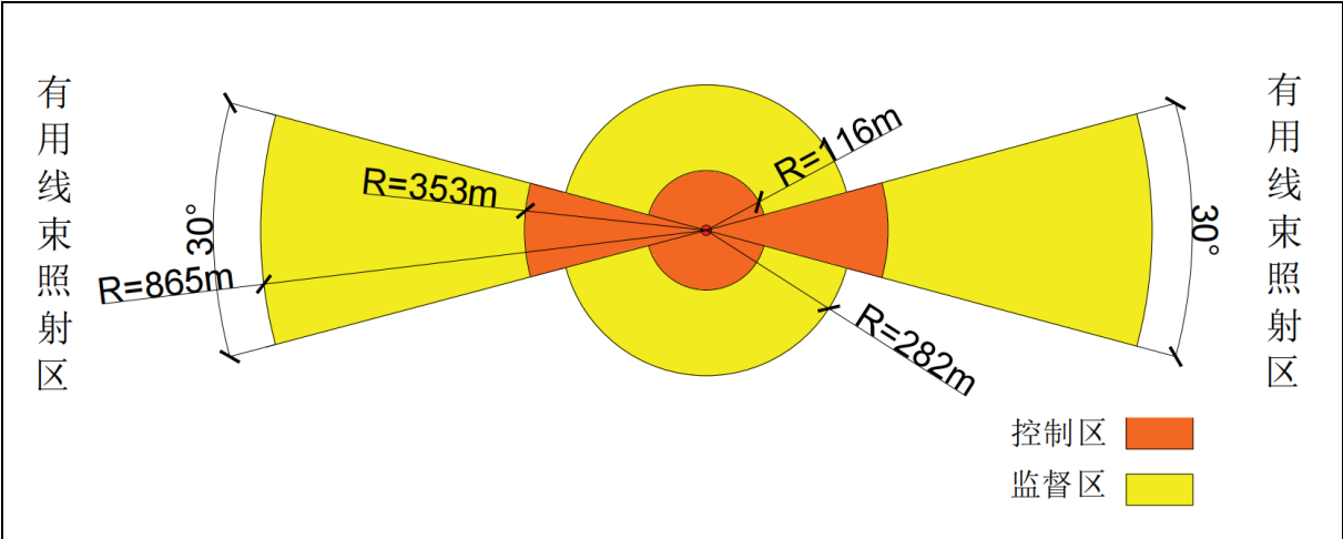
图 11-3 周向机分区示意图
