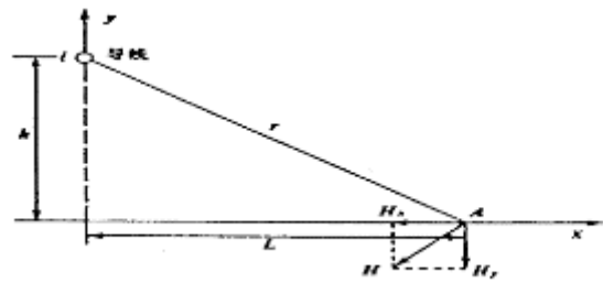
图 6-3 磁场向量图
