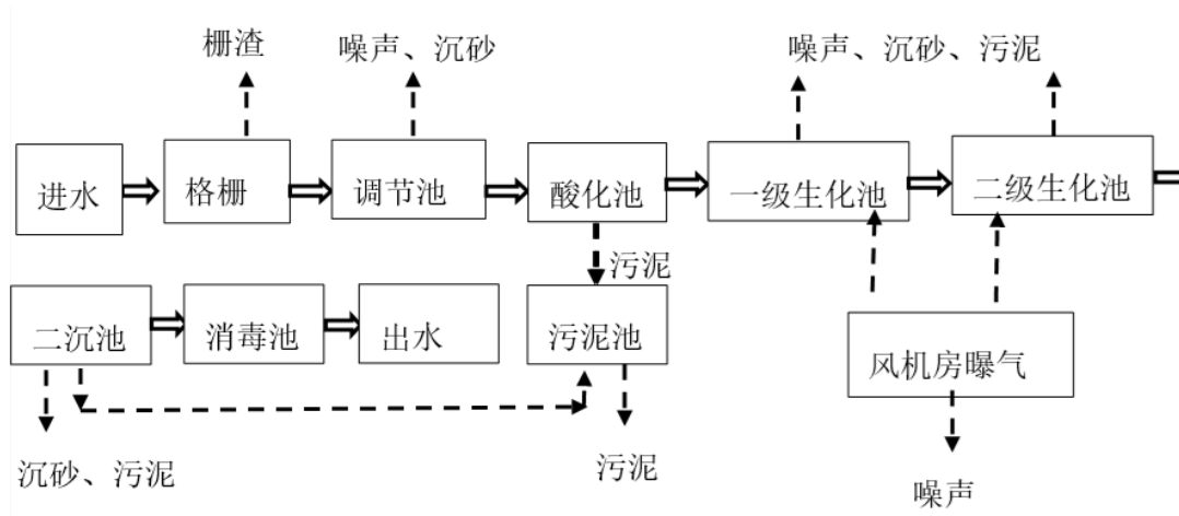
图 3.10-6 车河镇污水处理站生化处理工艺流程图
