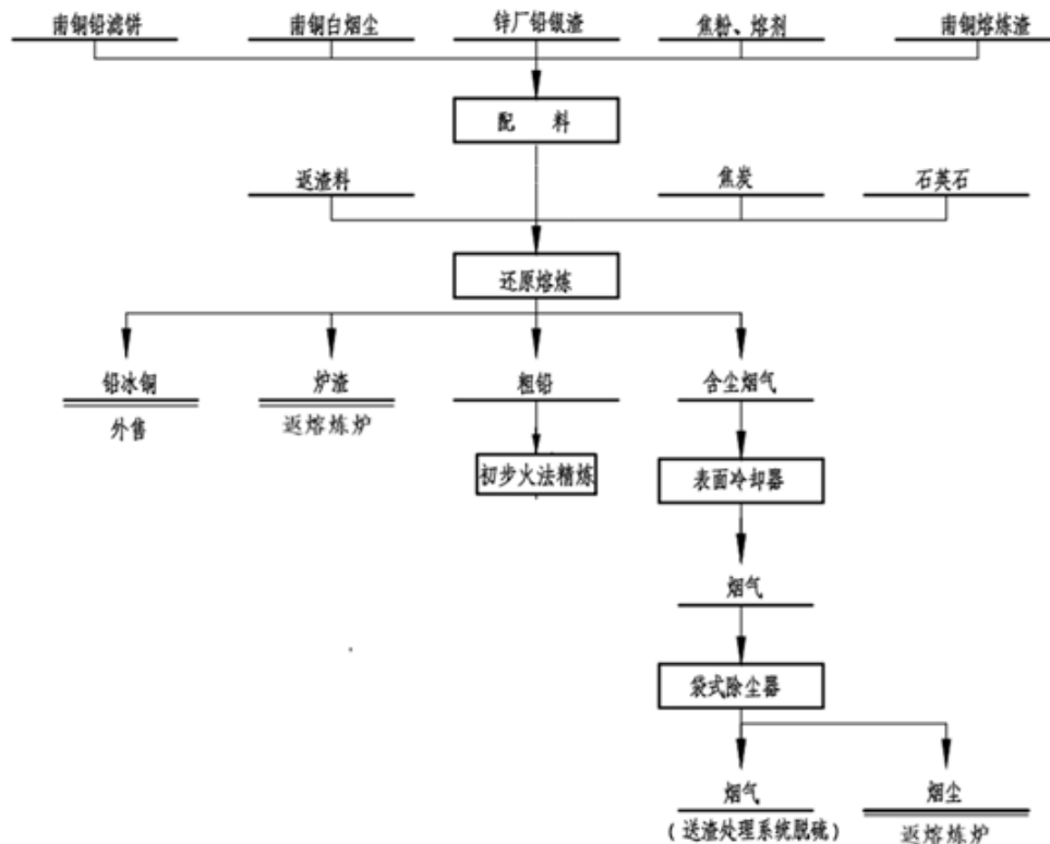
图 3.3-3 危废预处理工艺流程图
