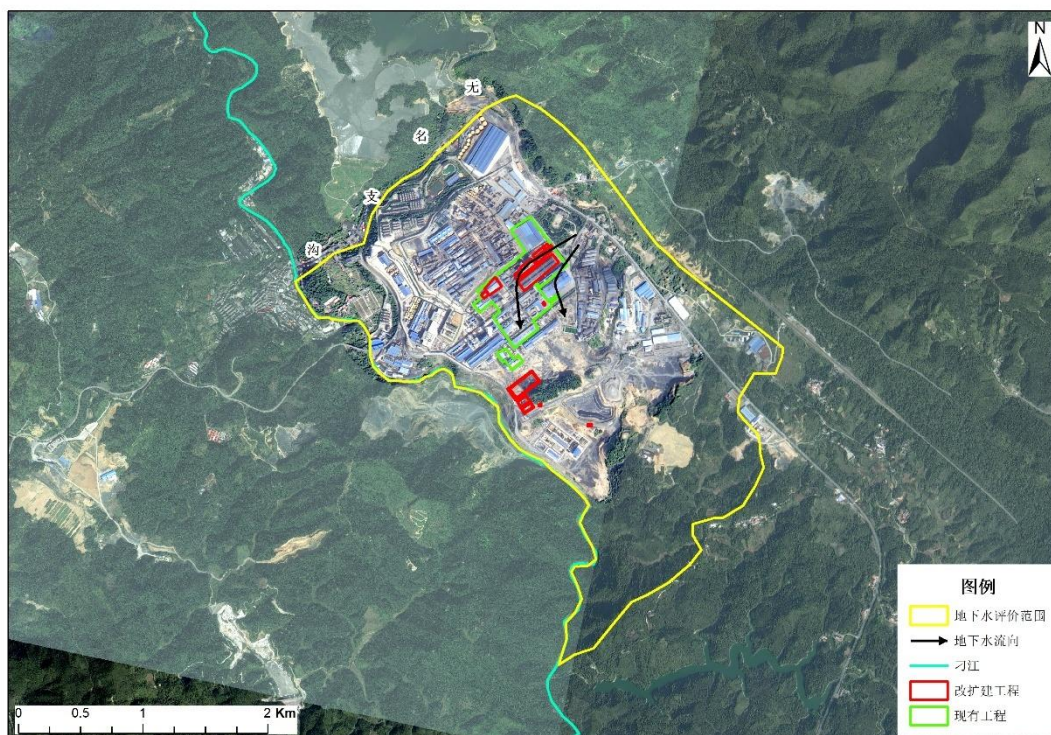
图 1.8-1 地下水评价范围图
