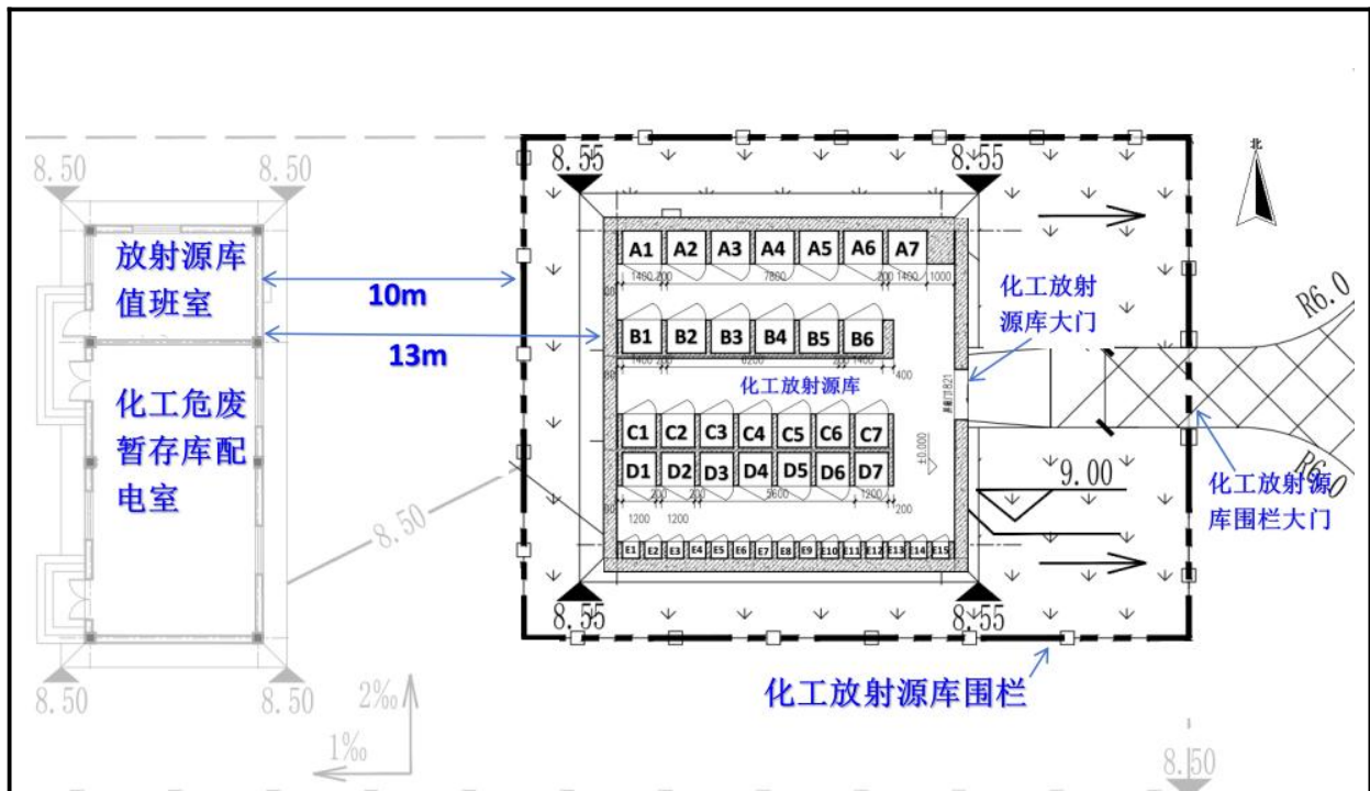
图 1-3 放射源库平面示意图
