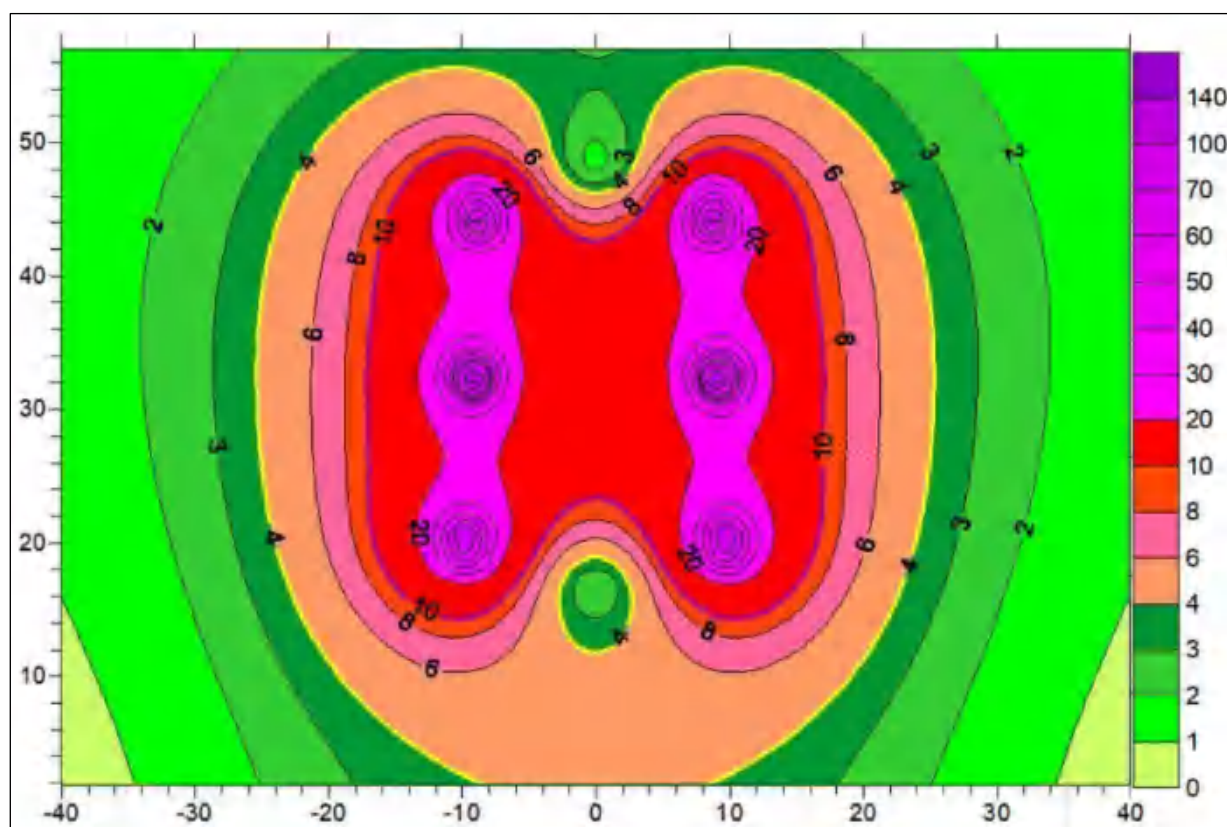
图 6-13 居民区导线对地 20m 工频电场强度空间分布等值线图 (kV/m)
