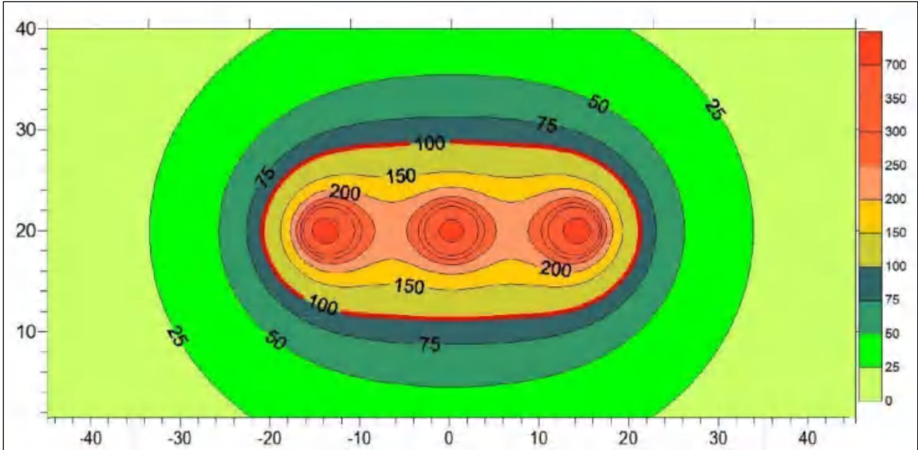
图 6-8 居民区导线对地 21m 工频磁场强度空间分布等值线图 (μT)
