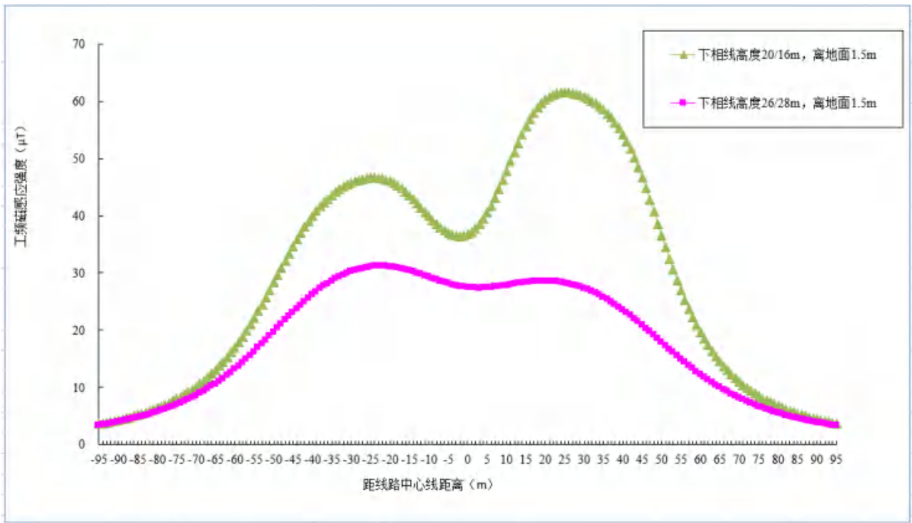
图 6-16 工频电场强度计算结果分布曲线图
