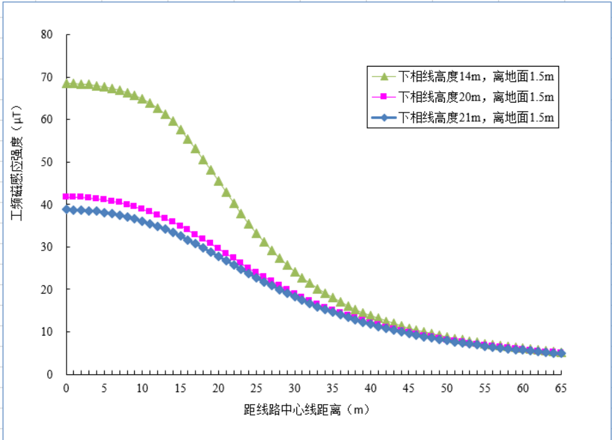
图 6-5 单回线路工频磁感应强度计算结果分布曲线图（居民区）
