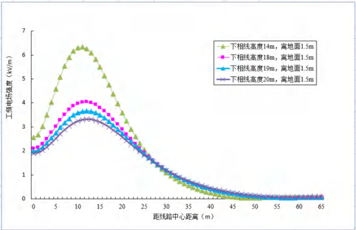
图 6-11 工频电场强度计算结果分布曲线图（居民区）
