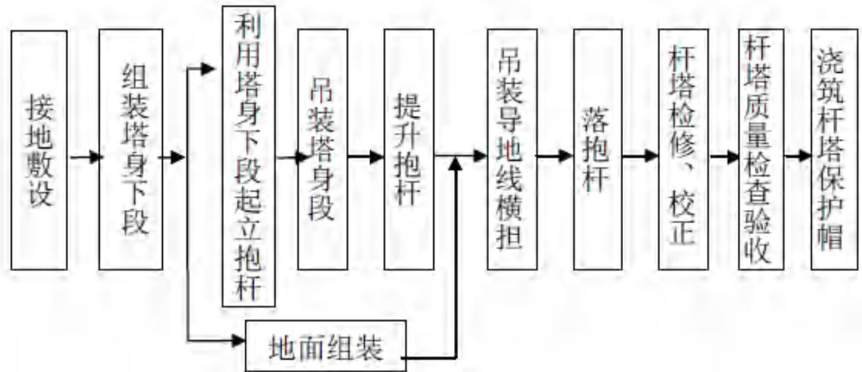
图 3-4 杆塔组立施工流程图
