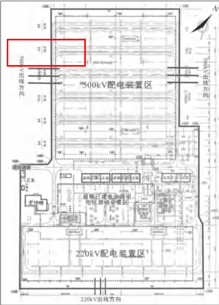
图 3-1 500kV 海港变电站间隔扩建区平面布置图
