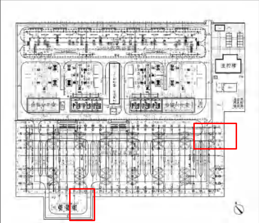
图3-2 500kV 民歌变电站间隔扩建区平面布置图
