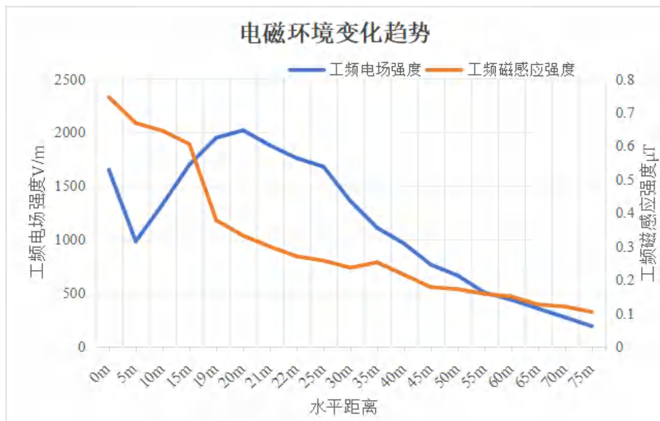
图 6-18 500kV 民邕甲线 (23#~24#) 跨越 500kV 南玉 I 线 (89#~90#) 衰减断面电磁环境变化趋势
