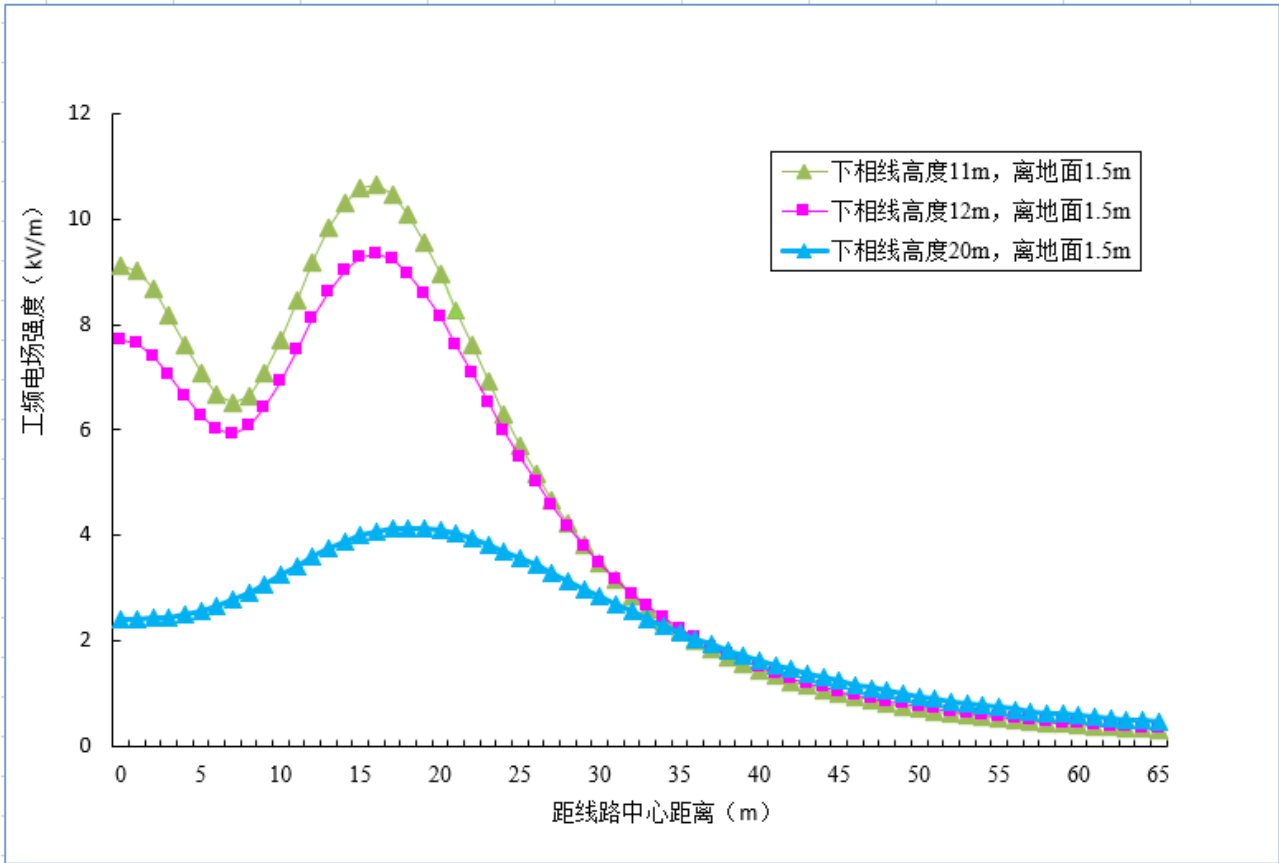
图 6-2 单回线路工频电场强度计算结果分布曲线图（非居民区）
