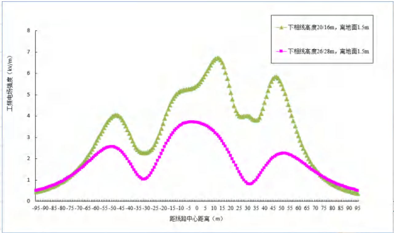
图 6-15 工频电场强度计算结果分布曲线图
