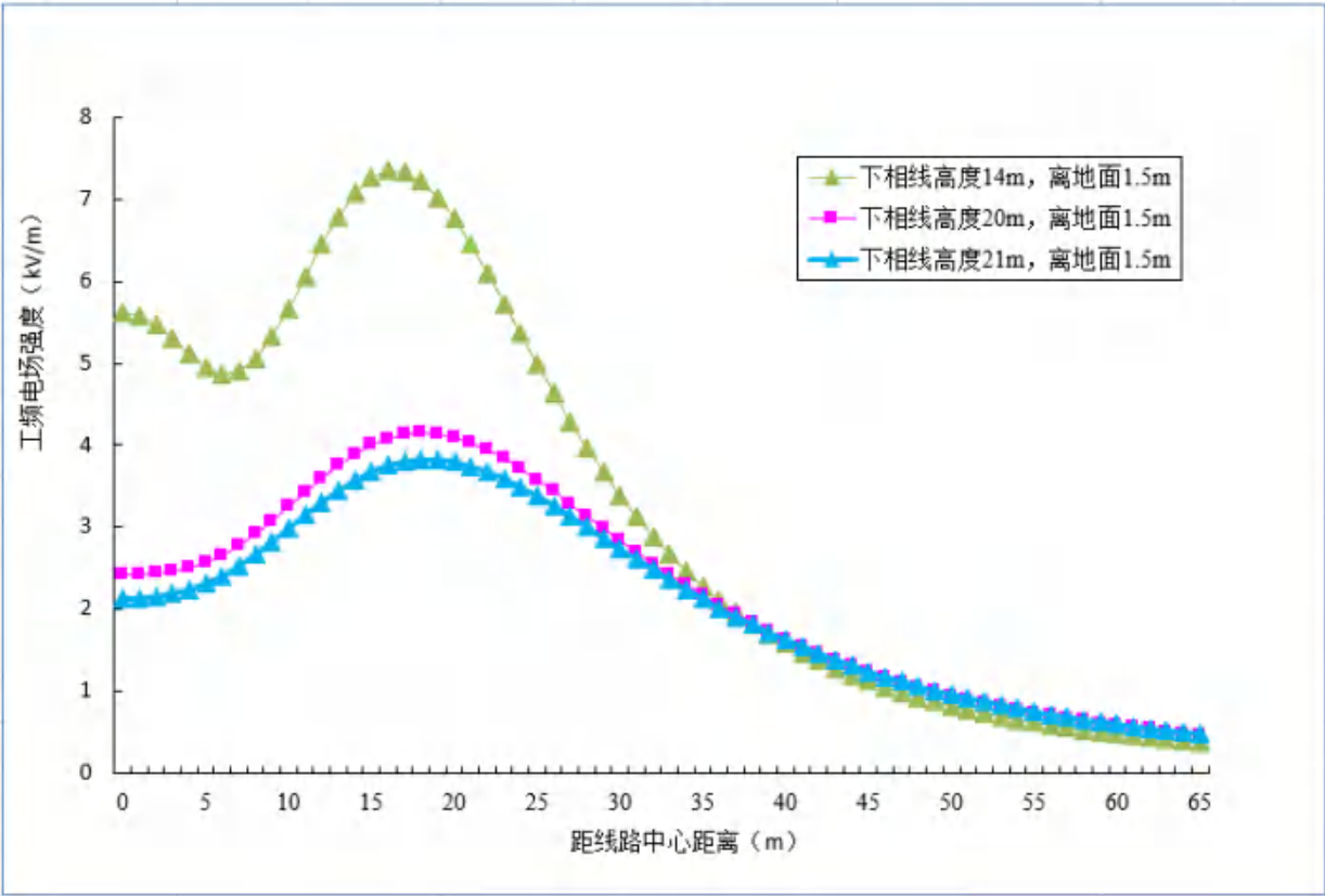
图 6-4 单回线路工频电场强度计算结果分布曲线图（居民区）
