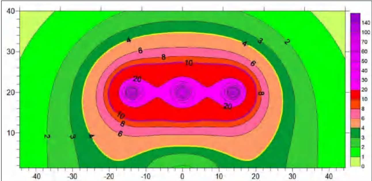
图 6-7 居民区导线对地 21m 工频电场强度空间分布等值线图 (kV/m)
