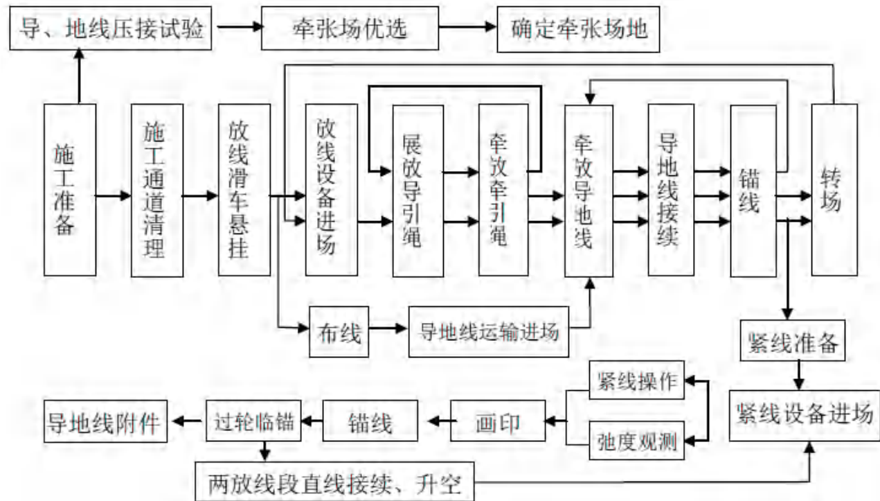
图 3-5 架线施工流程图
