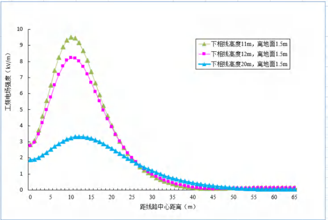
图 6-9 双回线路工频电场强度计算结果分布曲线图（非居民区）
