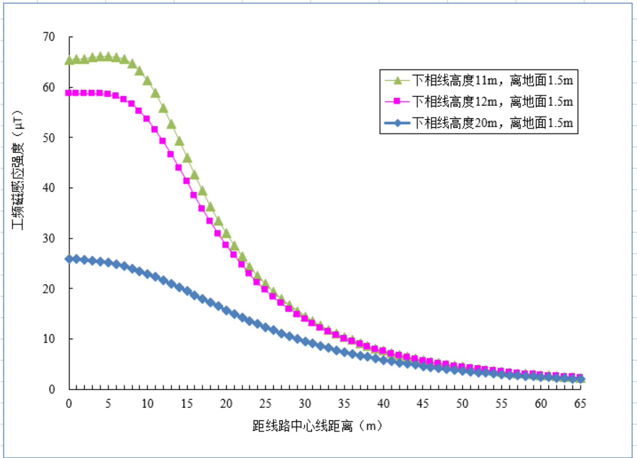
图 6-10 双回线路工频磁感应强度计算结果分布曲线图（非居民区）
