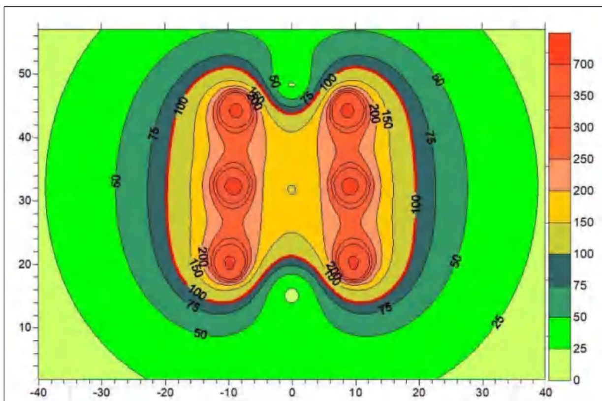
图 6-14 居民区导线对地 20m 工频磁感应强度空间分布等值线图 ( \mu\text{T} )
