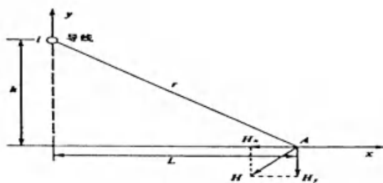
图 6-1 磁场向量图
