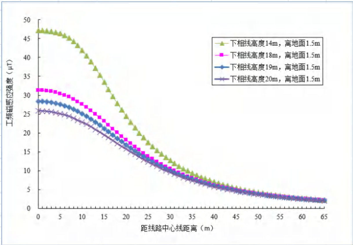
图 6-12 工频磁感应强度计算结果分布曲线图（居民区）
