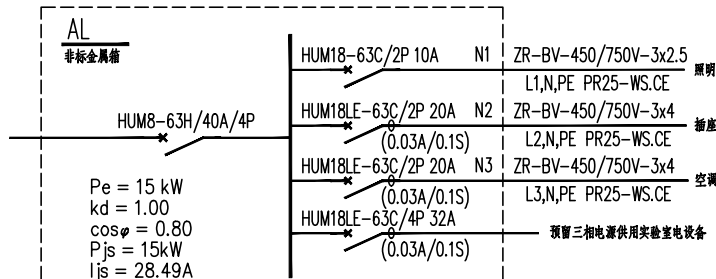
AL开关盒配电系统图
