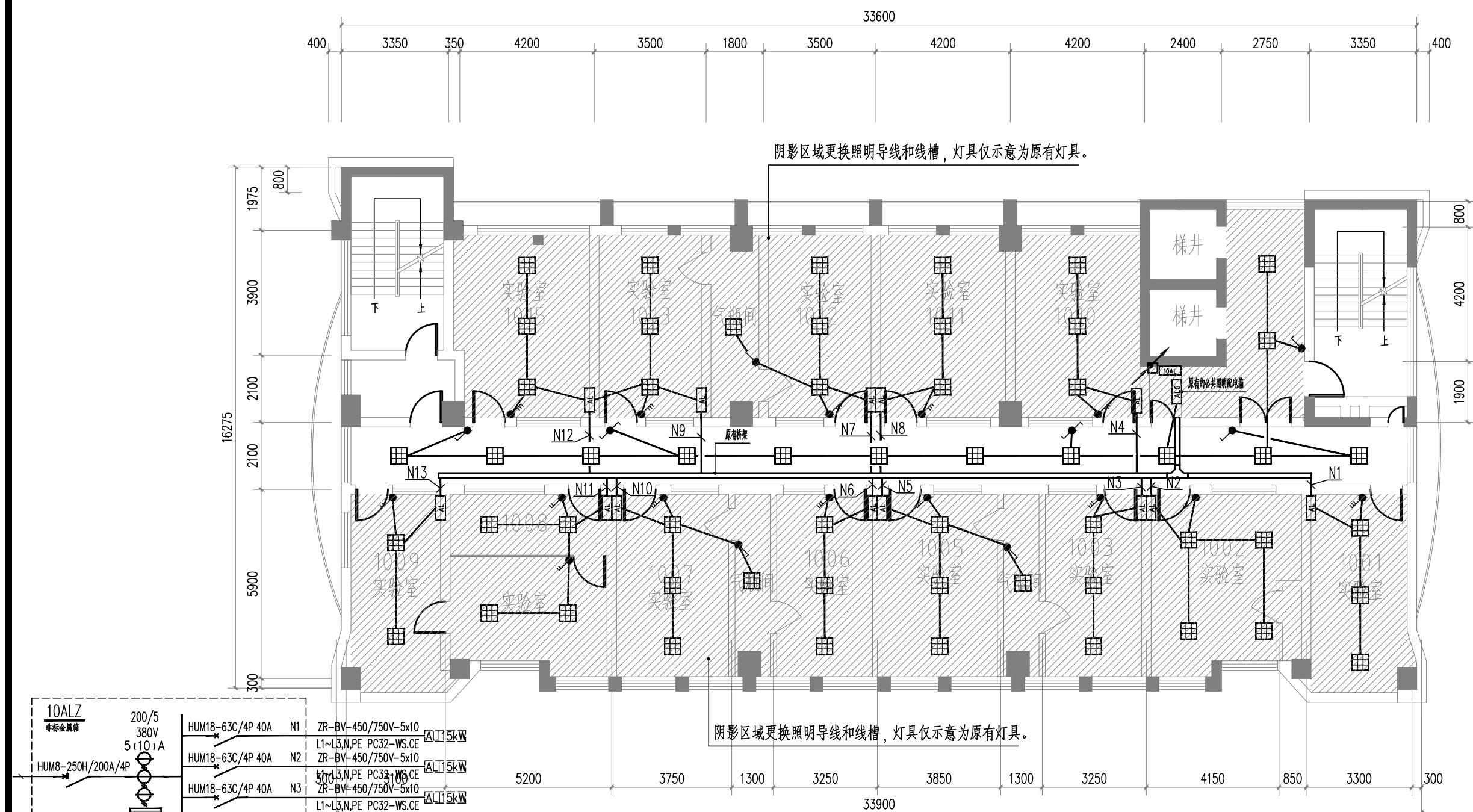
十层照明平面图 1:100 说明: 更换本层走廊灯盘20W, 及本层照明导线和线槽(包含走廊、实验室)。
