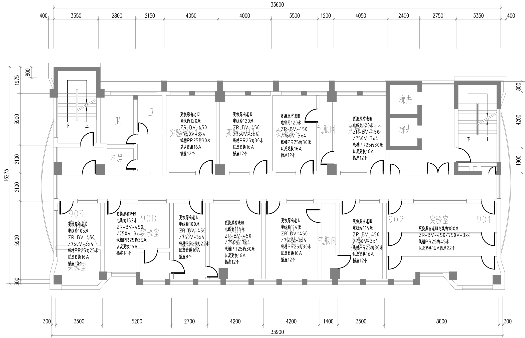
九层插座平面图 1:100
