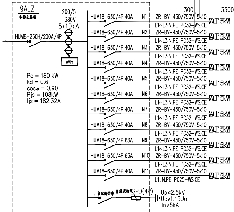
九层总配电箱系统图
