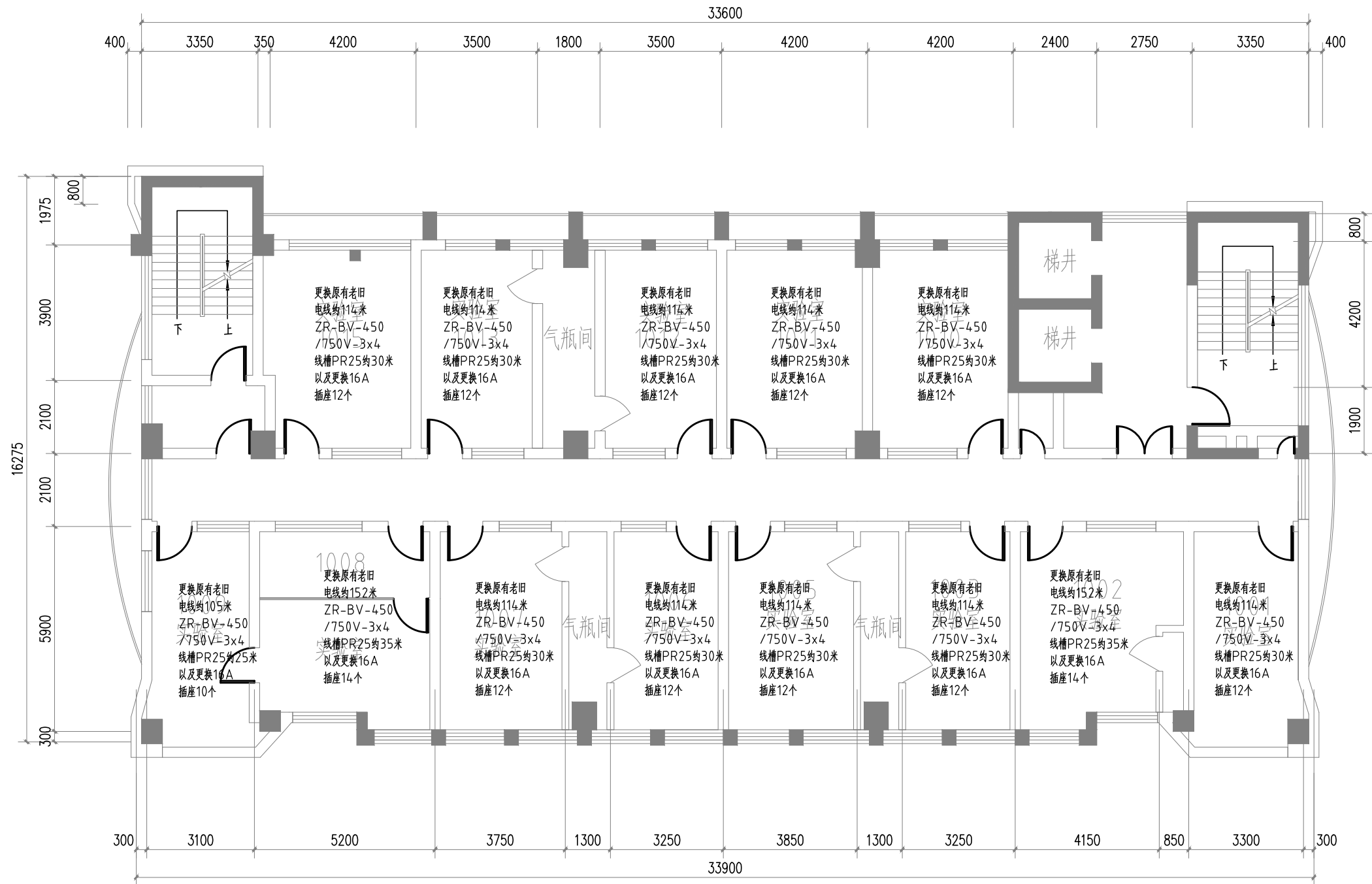
十层插座平面图 1:100
