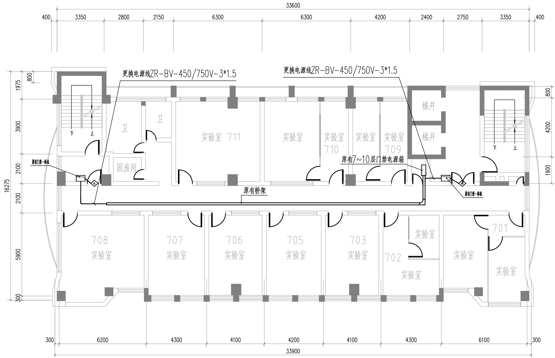
七~十层门禁平面图 1:100
